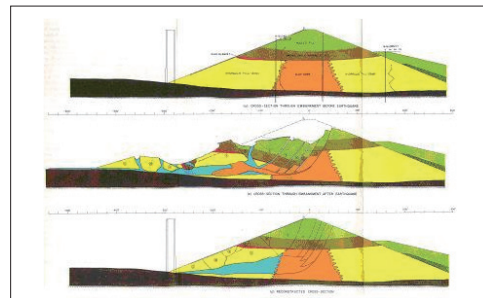
▲サンフェルナンド地震で崩壊したフィルダム
