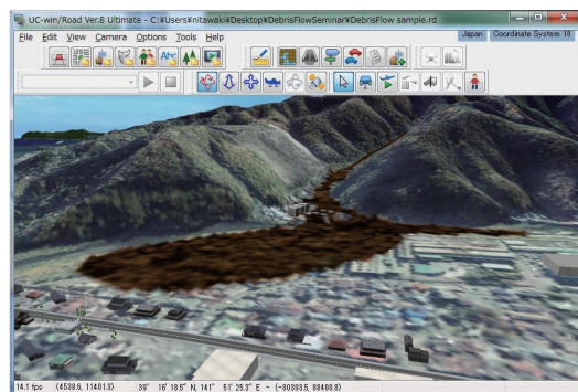
▲「UC-1 土石流シミュレーション」で見た解析結果(左)。その結果を UC-win/Road にインポートしたもの(右)は、土石流の流れと地形や街並みとの関係が分かりやすい
