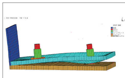
▲ NO TENSION 解析機能による解析例
