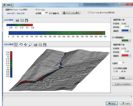
▲「UC-1 土石流シミュレーション」で見た解析結果(左)。その結果を UC-win/Road にインポートしたもの(右)は、土石流の流れと地形や街並みとの関係が分かりやすい
