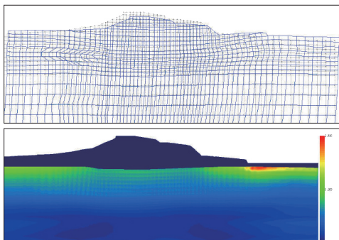
▲ UWLC による盛土の動的有効応力解析結果。 上が変位、下が過剰間隙水圧の分布図
